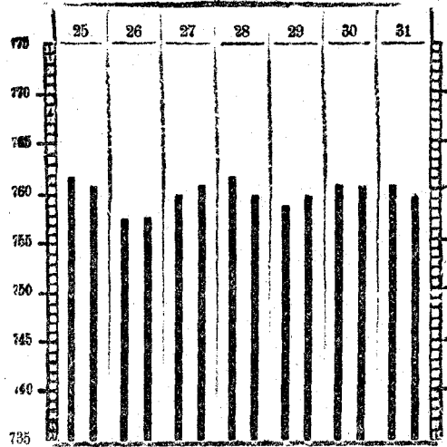
Alturas barométricas en Barcelona MAYO
